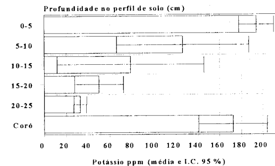
Fig. 6. Teores de potássio em camadas no perfil de solo e em câmaras de larvas do coró Diloboderus abderus . (Gassen e Kochhann, 1993).
