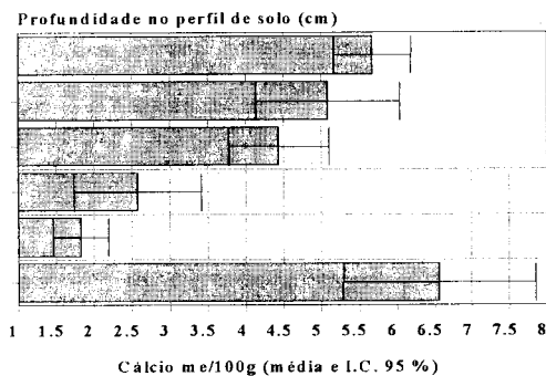
Fig. 3. Teores de cálcio em camadas no perfil de solo e em câmaras de larvas do coró Diloboderus abderus . (Gassen e Kochhann, 1993).
