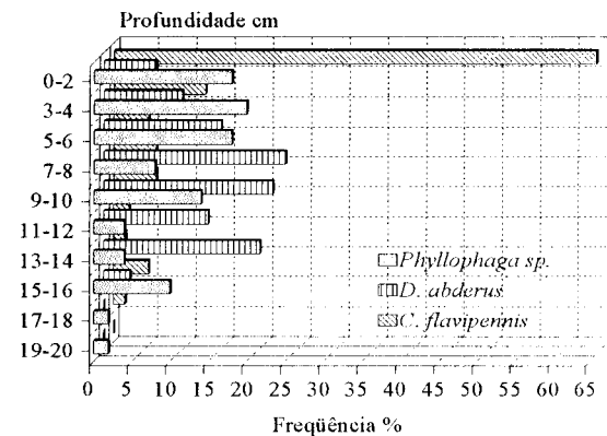
Fig. 7. Relação entre a profundidade (cm) no perfil do solo e a frequência de larvas de Diloboderus abderus , de Phyllophaga sp. e de Cyclocephala flavipennis , coletadas em lavoura de soja, após a colheita, durante o mês de abril (Gassen, 1993a).
