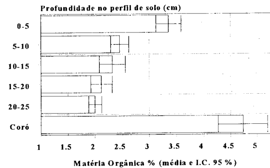
Fig. 5. Teores de matéria orgânica em camadas no perfil de solo e em câmaras de larvas do coró Diloboderus abderus . (Gassen e Kochhann, 1993).
