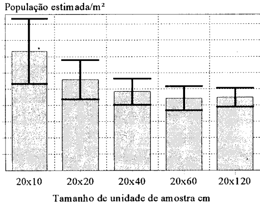
Fig. 13. Estimativas de população de larvas de Diloboderus abderus , sob diferentes tamanhos de unidade de amostra (I.C. 95 %) (Gassen, 1992a,c).
