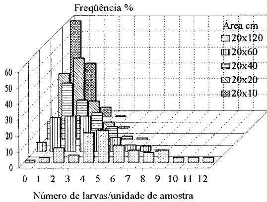
Fig. 14. Relação entre a frequência (%) de larvas de Diloboderus abderus e diferentes tamanhos de unidades de amostra (área cm 2 ) em lavoura de trigo sob plantio direto (Gassen e Corseuil, 1993).
