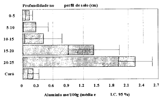
Fig. 2. Teores de alumínio em camadas no perfil de solo e em câmaras de larvas do coró Diloboderus abderus . (Gassen e Kochhann, 1993).
