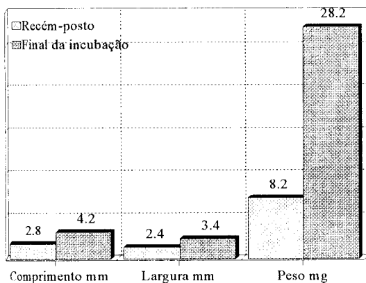
Fig. 5. Tamanho e peso de ovos de Diloboderus abderus durante a incubação (Gassen e Schneider, 1992).
